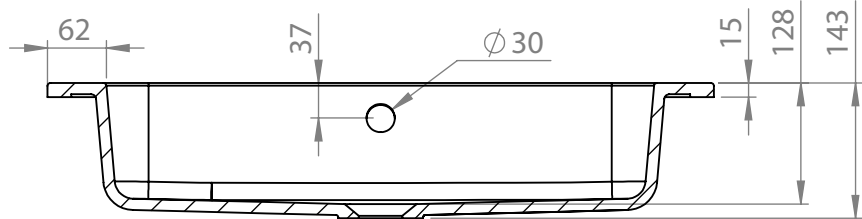
PRZEKRÓJ N-N SKALA 1 : 8
