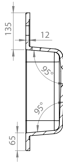
PRZEKRÓJ M-M SKALA 1 : 8
